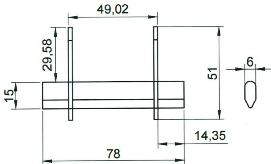
Zīmējums 3.1. NH00 Drošinātāja nazis
