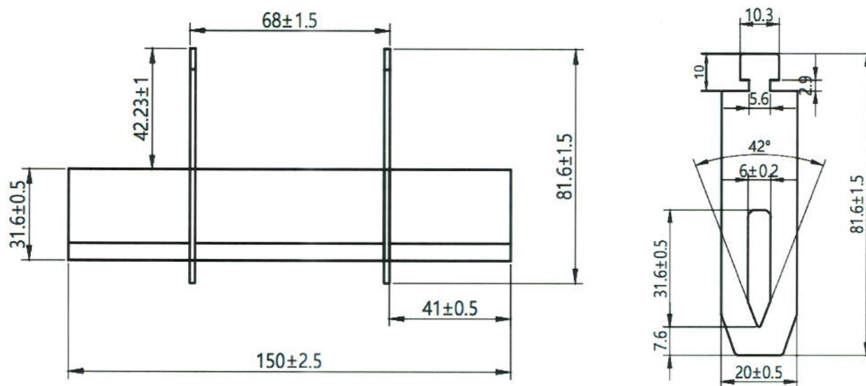
Zīmējums 3.4 NH3 Drošinātāja nazis
