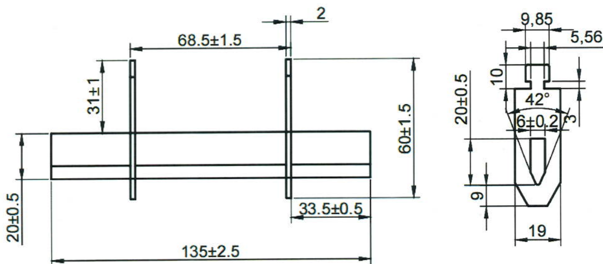
Zīmējums 3.2 NH1 Drošinātāja nazis
